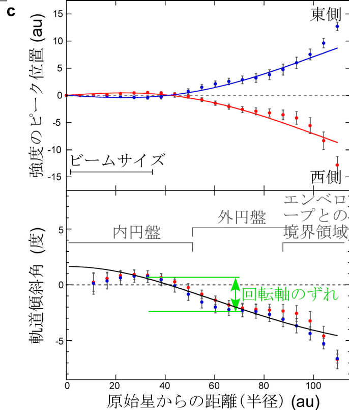
図1 原始星 IRAS04368+2557 周りの初期円盤のアルマ望遠鏡による観測結果
